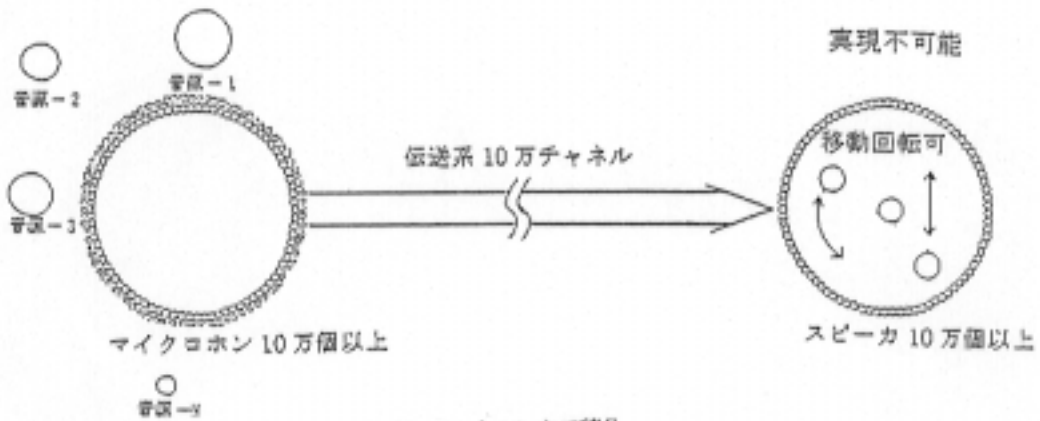
図-2 キルヒホフ積分
